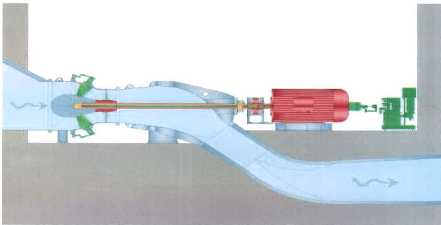
Slika – Kaplan turbine
